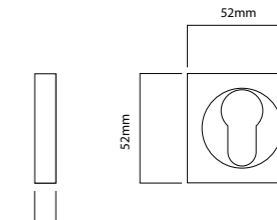
EURO ESCUTCHEONS SQUARE
