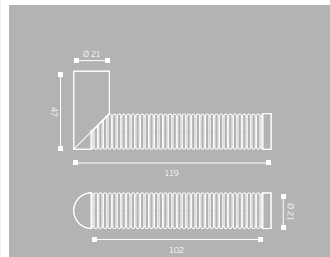
IN.00.441.RB08M Puxador de porta com roseta. Material: EN 1.4301 + Silver 925 / Lever handle with rose for doors./ Manilla con roseta para puertas.
