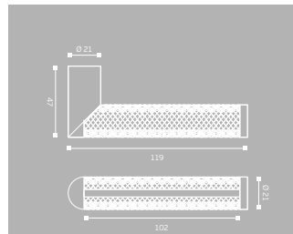
IN.00.440.RB08M Puxador de porta com roseta. Material: EN 1.4301 + Silver 925 / Lever handle with rose for doors./ Manilla con roseta para puertas.
