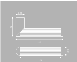
IN.00.442.RB08M Puxador de porta com roseta. Material: EN 1.4301 + Silver 925 / Lever handle with rose for doors./ Manilla con roseta para puertas.
