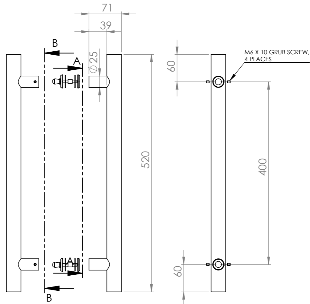
SECTION A-A
